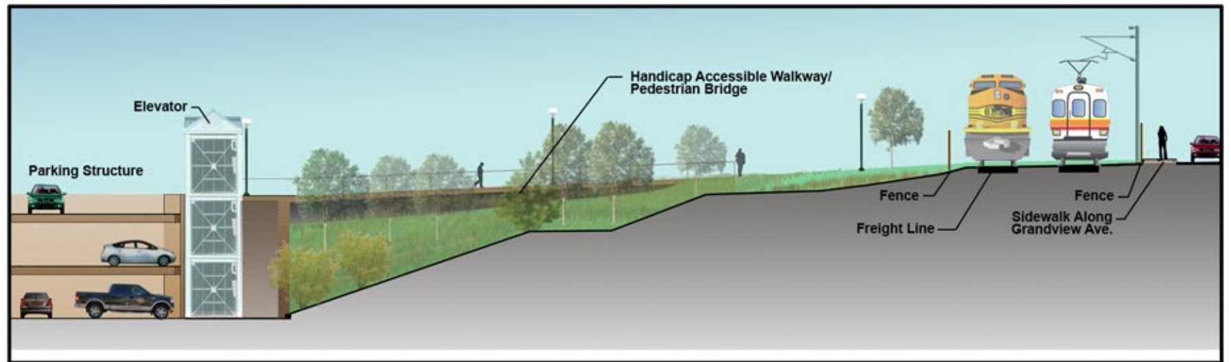
Section D-D
