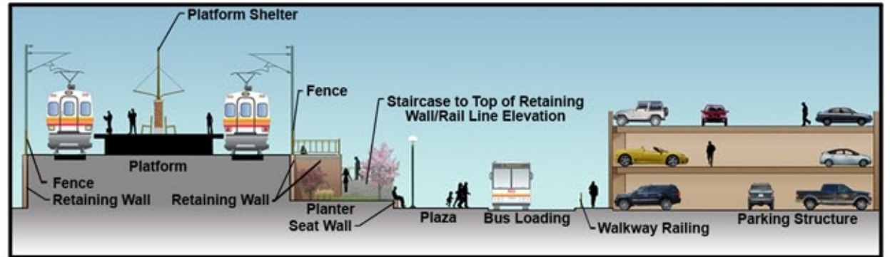
Section D-D
